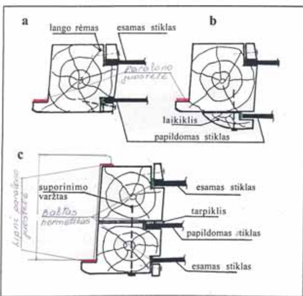
Brėžinys Nr. 1. Lango papildomo ištiklinimo pavyzdžiai
